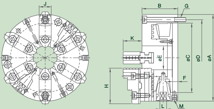
尺寸圖 » Dimensions
