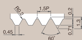
Pitch 1.5 齒型詳圖
