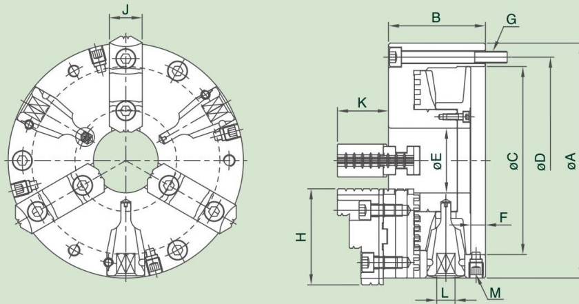
尺寸圖 » Dimensions
